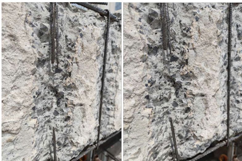
Fotografías 5 y 6. Vista de la rotura de estribos evidenciada durante los trabajos de escarificado de la zona dañada por corrosión.
